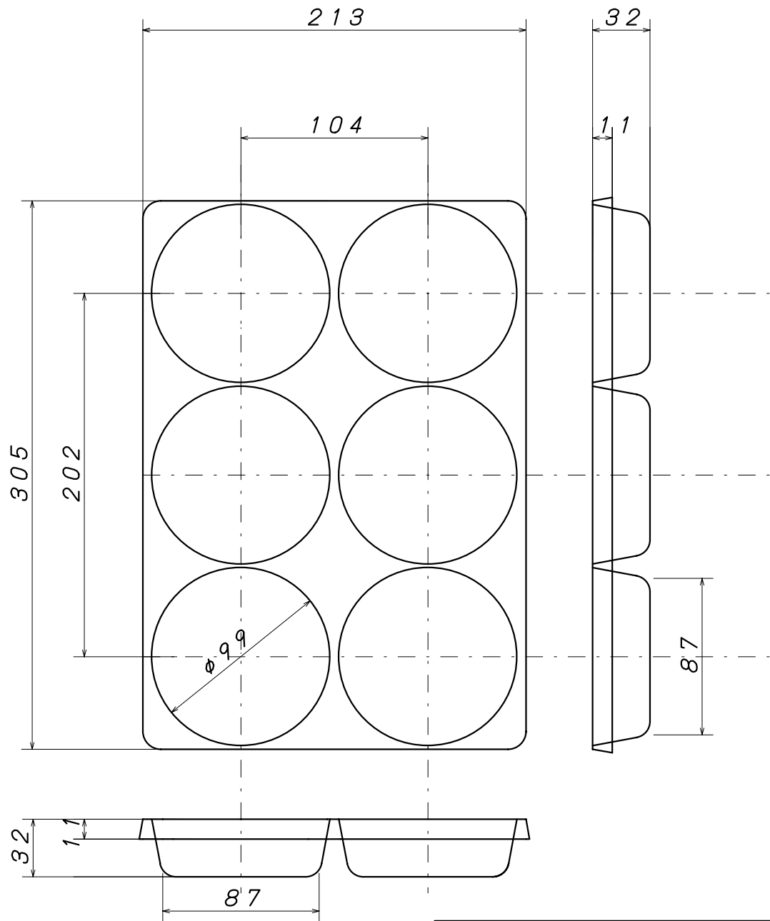
工業用トレイ製品寸法図
